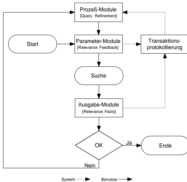
Abb. 2. Schnittstellen-Module und ihre Verknüpfung
